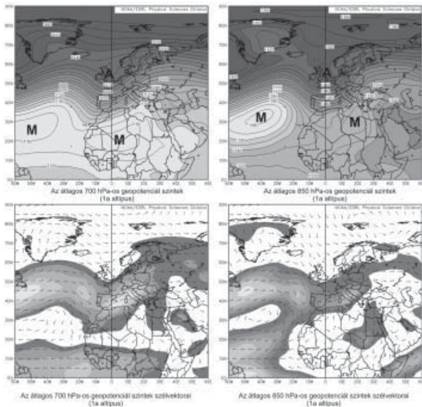
4. ábra: Az 1a altípus 60 eseményének átlagos AT-térképei és szélvektorai Figure 4.: The average geopotential height and wind vector maps of the 60 type-1a episodes
