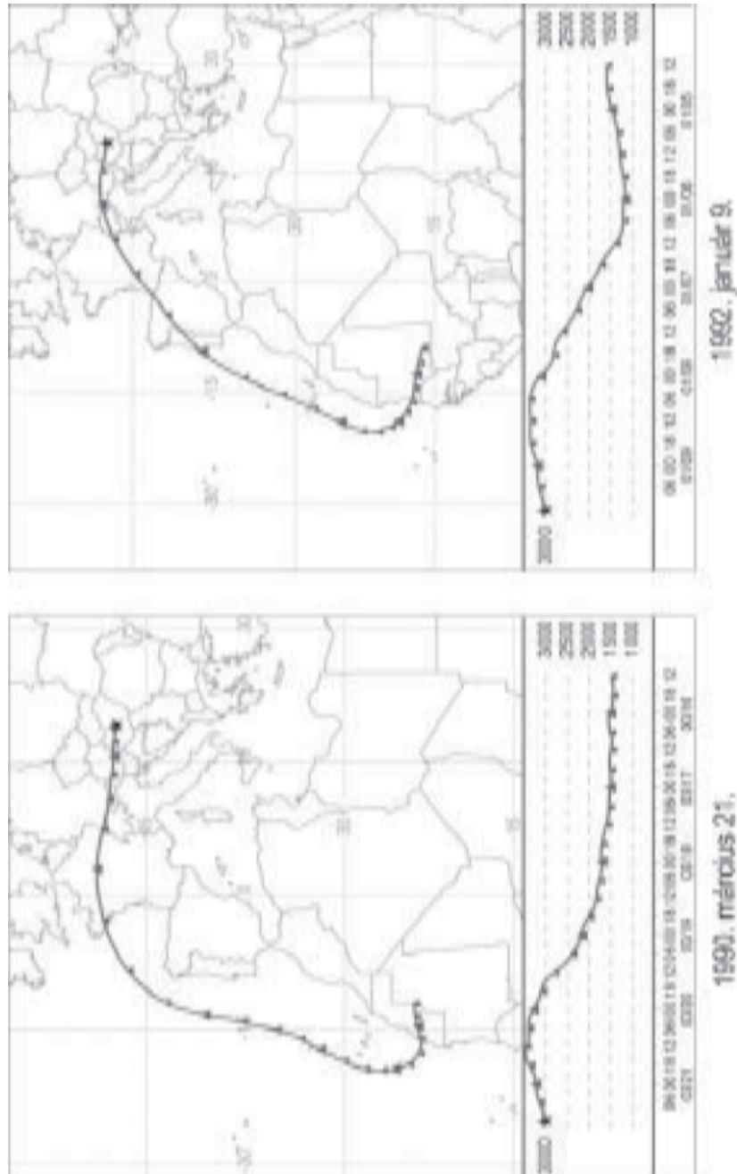
9. ábra: A 3-as típusú poros esemény jellemző szállítási útvonala Figure 9.: Typical air mass trajectories of type-3 episodes
