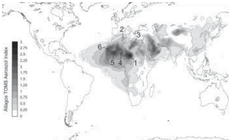
1. ábra: Az 1979–2009 közötti időszak adatszolgáltatási és mérési hibáktól mentes 23 teljes évének napi TOMS Aeroszol Indexeiből szerkesztett globális átlag-térkép (a számok a legfontosabb észak-afrikai forrásterületeket jelölik – lásd később a szövegben)
