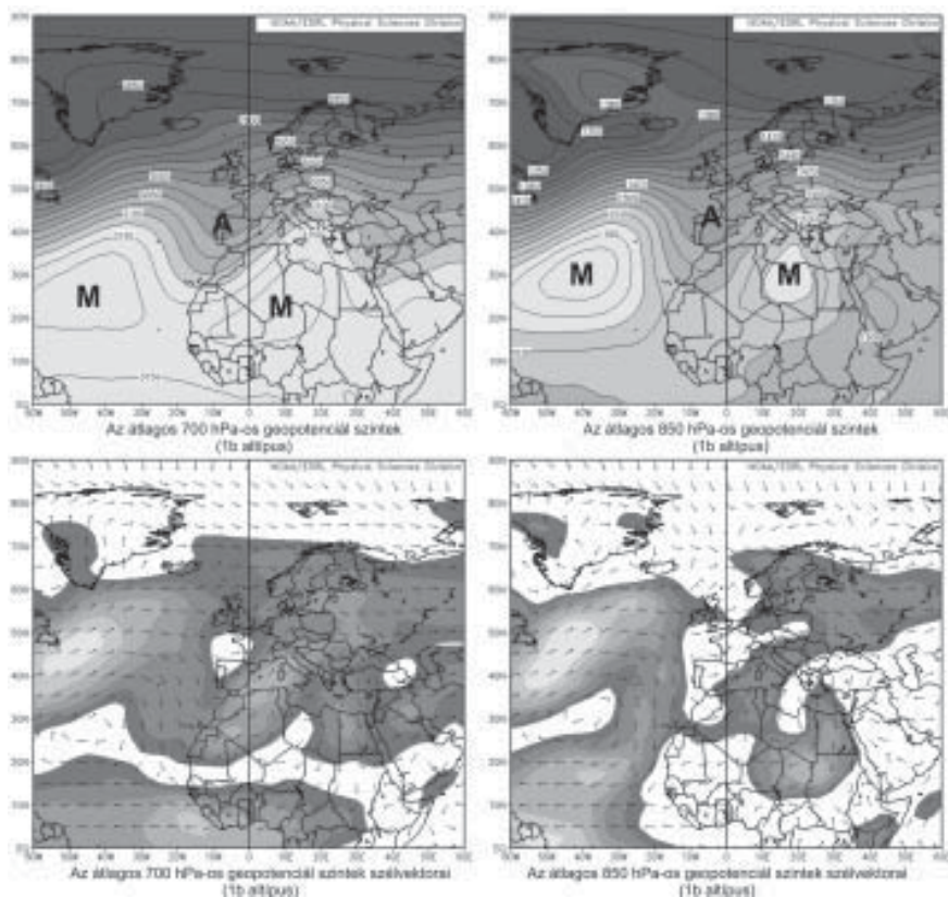
5. ábra: Az 1b altípus 21 eseményének átlagos AT-térképei és szélvektorai Figure 5.: The average geopotential height and wind vector maps of the 21 type-1b episodes
