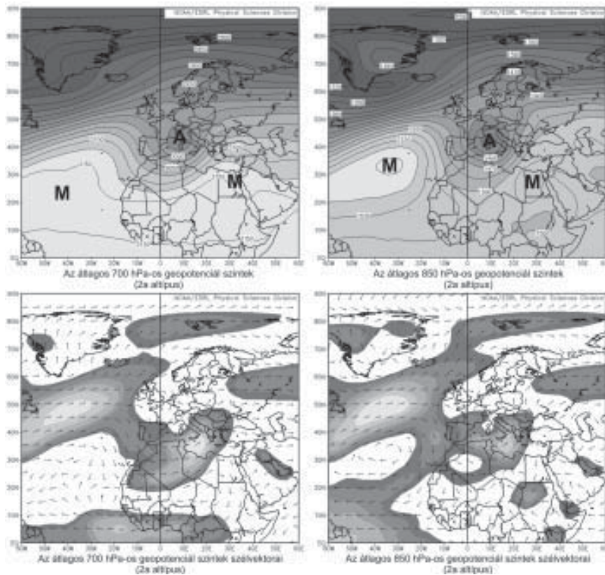
6. ábra: A 2a altípus 31 eseményének átlagos AT-térképei és szélvektora Figure 6.: The average geopotential height and wind vector maps of the 31 type-2a episodes
