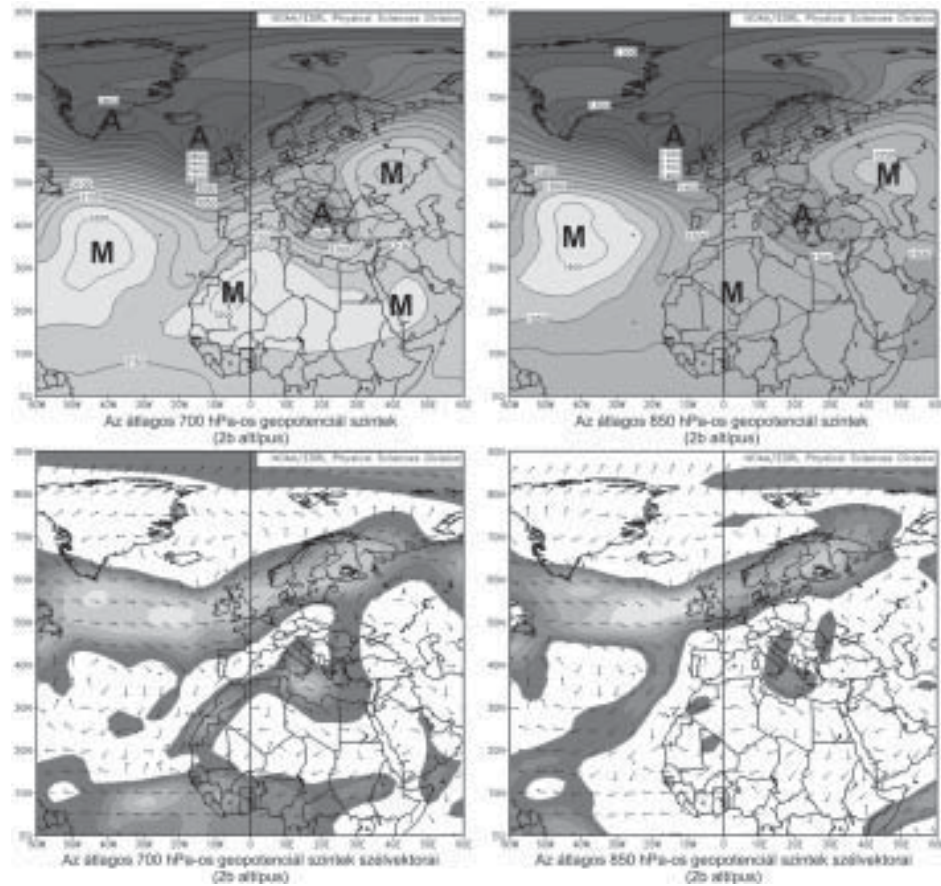
7. ábra: A 2b altípus 2 eseményének átlagos AT-térképei és szélvektorai Figure 7.: The average geopotential height and wind vector maps of the 2 type-2b episodes
